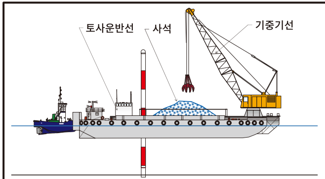
투입 장소 부근에서 토사운반선을 기중기선에 접현시켜 운반한 사석을 환적합니다.
