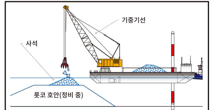
환적한 사석은 기중기선을 이용하여 직접 투입 위치에 투입합니다.
