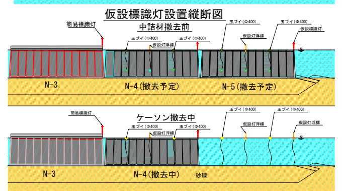
仮設標識灯および仮設灯浮標設置概要図
