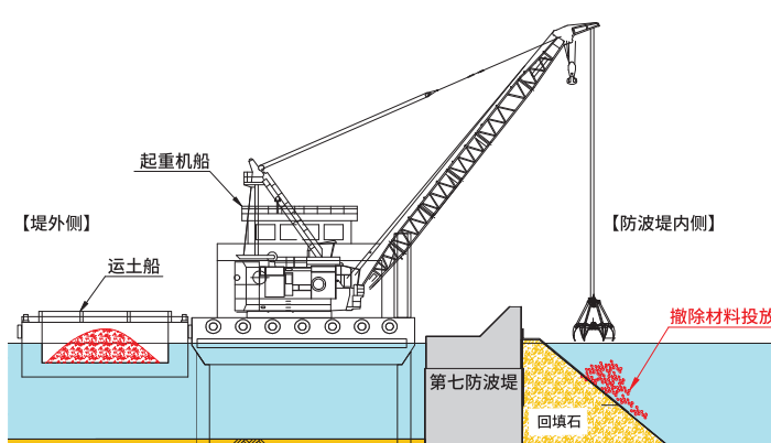
撤除材料投放样子(第七防波堤)
