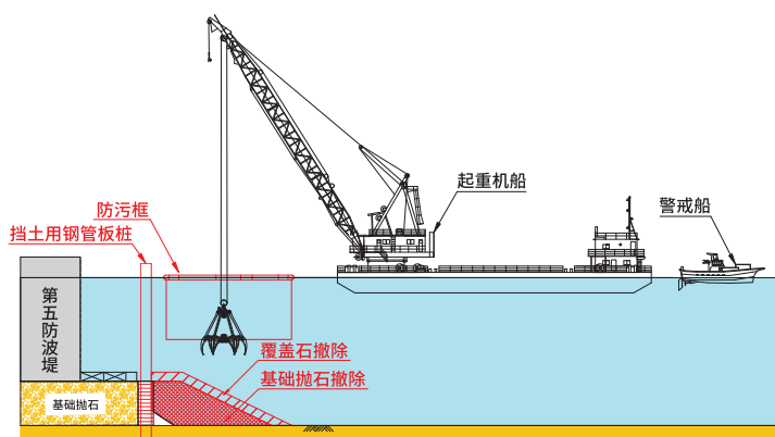
构筑物拆除工程与附带工程
