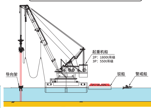
钢管板桩与钢管桩打设样子(共通)
