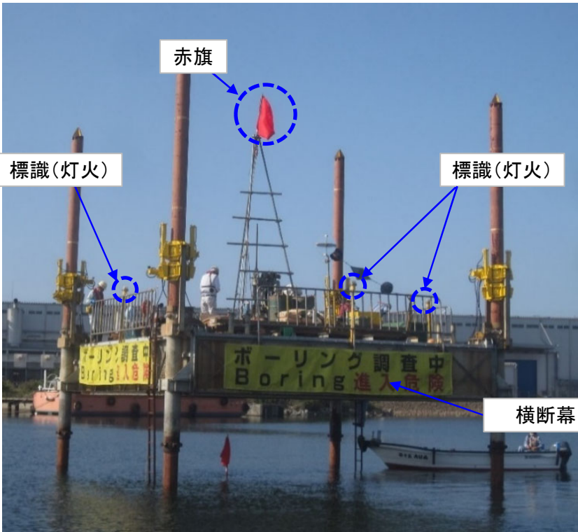
写真-3.1 スパット台船設置状況
