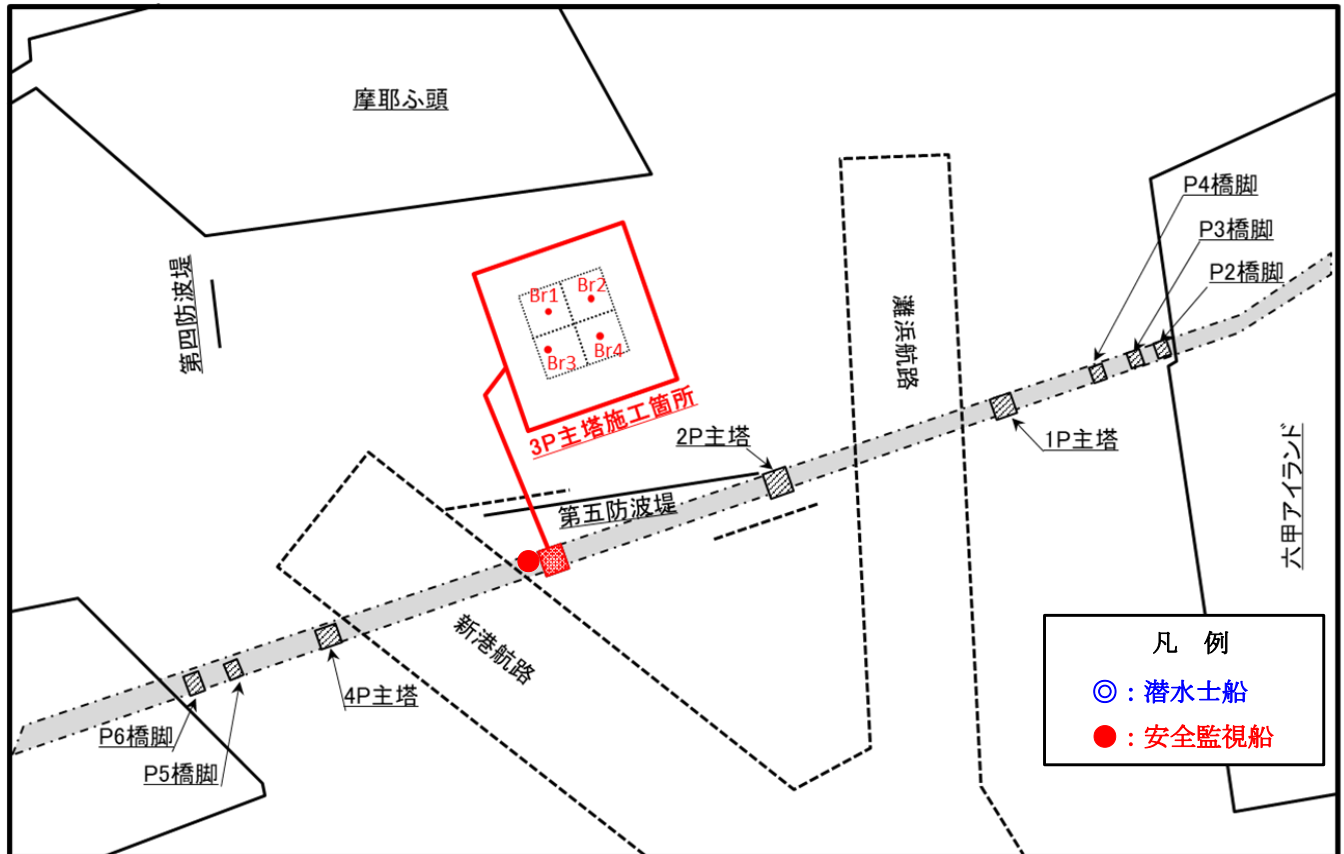
ボーリング調査略図
